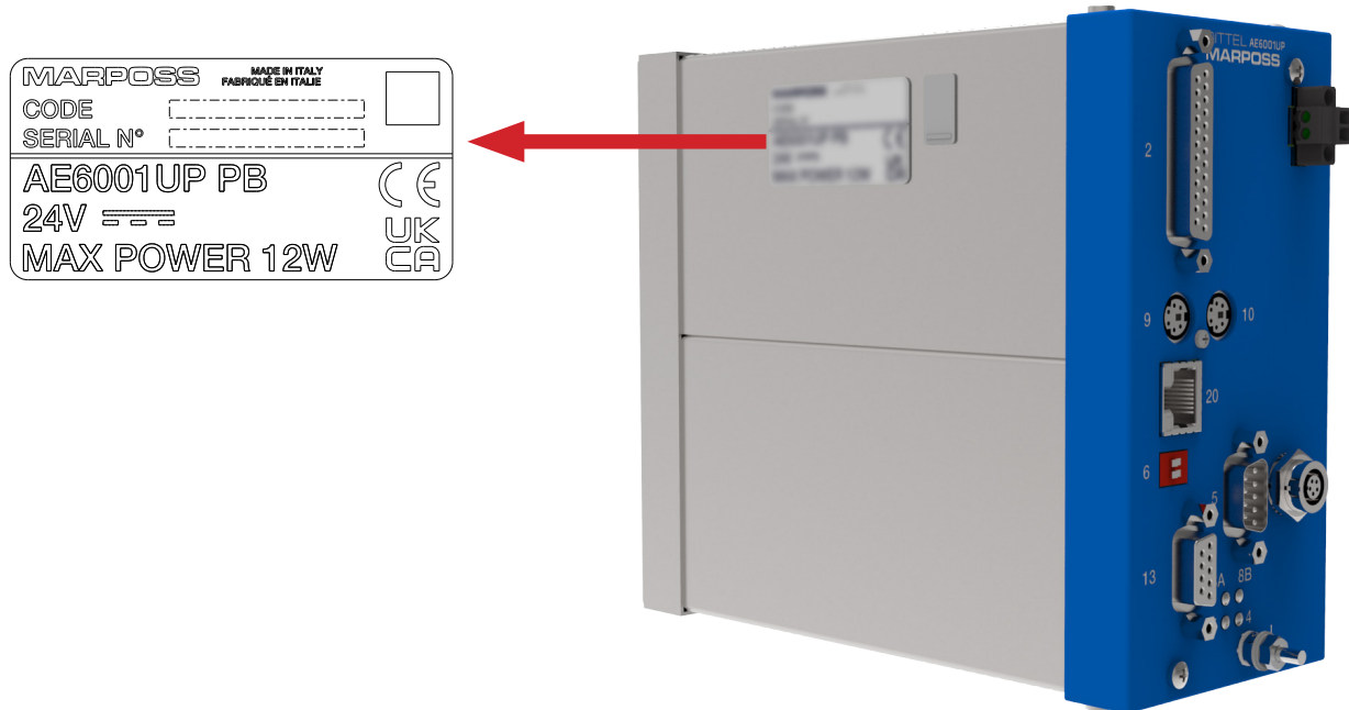
Fig.1. AE6001 UP Posizione della targhetta dati
