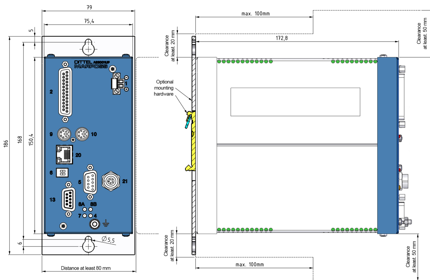
Fig.8. Esempio di montaggio di AE6001 UP su una guida DIN
