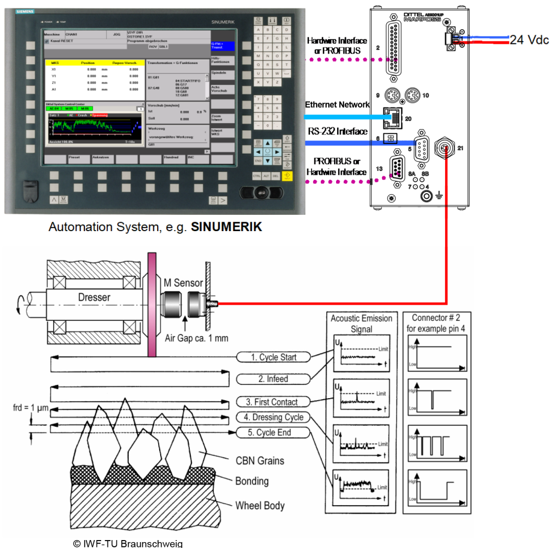
Fig.4. Esempio di sorveglianza di un ciclo di diamantatura mediante valutazione del segnale di emissione acustica (AE) su AE6001 UP PB
