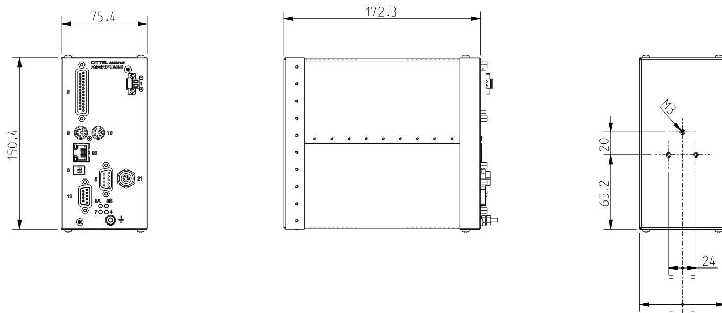
Fig.6. Dimensioni AE6001 UP
